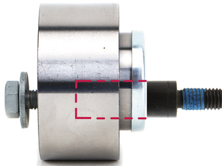
Obrázek 4: Napínací kladka INA s objímkou a upevňovacím šroubem v montážní poloze
