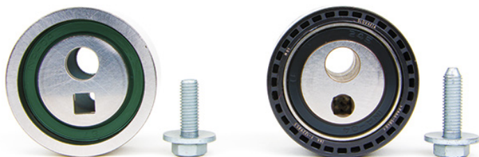
Obrázek 2: 531 0780 10 - napínací kladka INA s přiloženým šroubem
