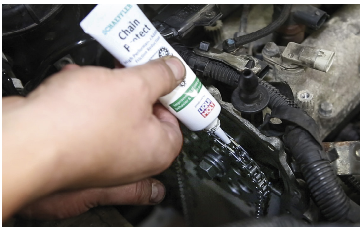
Obrázek 2: Aditivum Chain Protect od společnosti Schaeffler se nanese během montáže řetězu na všechny komponenty řetězového pohonu
