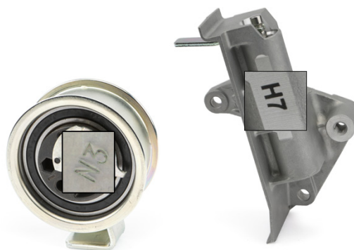
Obrázek 1: Napínací kladka 531 0396 20 s tlumičem vibrací 533 0039 10
